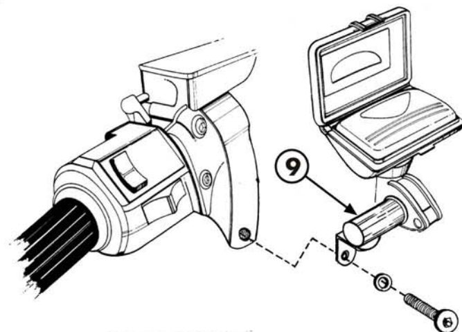
FISSAGGIO CON ART. Z278 (adattatore per manubri non tondi ) FIXING WITH ITEM Z278 ( adaptator for non-round handlebars ) FIXAGE AVEC ART. Z278 ( adaptateur pour guidons pas ronde )
